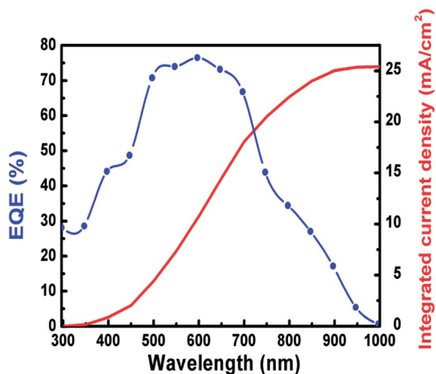
Fig. 7 EQE spectrum.
