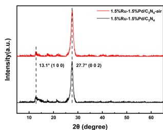
Fig. 2 XRD patterns of 1.5\%Ru-1.5\%Pd/C_3N_4 and 1.5\%Ru-1.5\%Pd/C_3N_4 -air.
