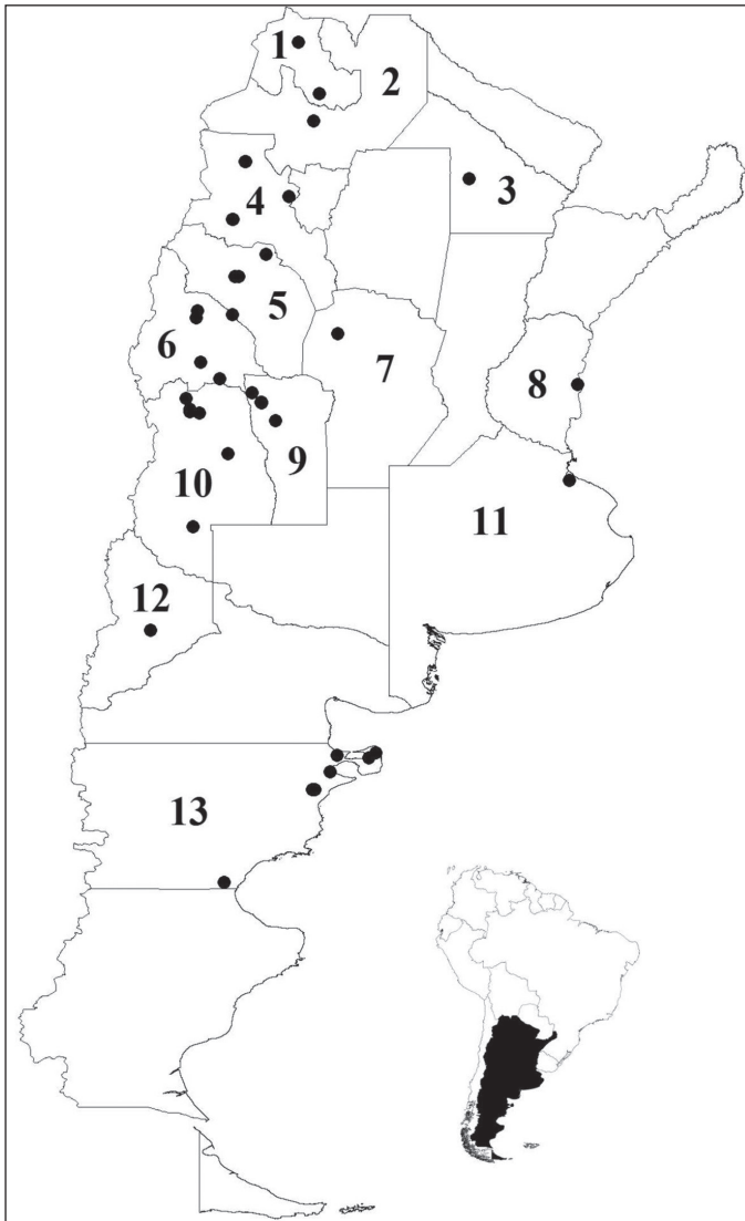
Figure 23. Geographical distribution of sixteen species of Histeridae in Argentina. Provinces: 1 Jujuy: Euspilotus (Hesperosaprinus) caesopygus , E. (s. str.) lacordairei , E. (s. str.) lepidus 2 Salta: E. (H.) caesopygus , E. (H.) strobeli 3 Chaco: E. (s. str.) lacordairei 4 Catamarca: E. (H.) caesopygus , E. (H.) pavidus , E. (s. str.) lacordairei , E. (s. str.) richteri 5 La Rioja: E. (H.) caesopygus , E. (s. str.) lacordairei , E. (s. str.) lepidus , E. (s. str.) richteri 6 San Juan: E. (H.) modestus , E. (H.) parenthesis , E. (H.) pavidus , E. (s. str.) lacordairei , E. (s. str.) ornatus , Xerosaprinus (Xerosaprinus) diptychus 7 Córdoba: E. (H.) pavidus 8 Entre Ríos: E. (H.) pavidus 9 San Luis: E. (H.) caesopygus , E. (H.) pavidus , E. (s. str.) lacordairei , E. (s. str.) ornatus 10 Mendoza: Carcinops (s. str.) troglodytes , E. (H.) azureus , E. (H.) caesopygus , E. (H.) connectens , E. (H.) modestus , E. (H.) parenthesis , E. (H.) pavidus , E. (H.) strobeli , E. (s. str.) lacordairei , E. (s. str.) lepidus , E. (s. str.) ornatus , E. (s. str.) patagonicus , E. (s. str.) richteri , Hololepta (Leonota) reichii , Phelister rufinotus , Xerosaprinus diptychus 11 Buenos Aires: E. (s. str.) patagonicus 12 Neuquén: E. (s. str.) patagonicus 13 Chubut: C. (s. str.) troglodytes , E. (H.) modestus , E. (s. str.) lacordairei , E. (s. str.) ornatus , E. (s. str.) patagonicus , E. (s. str.) richteri .
