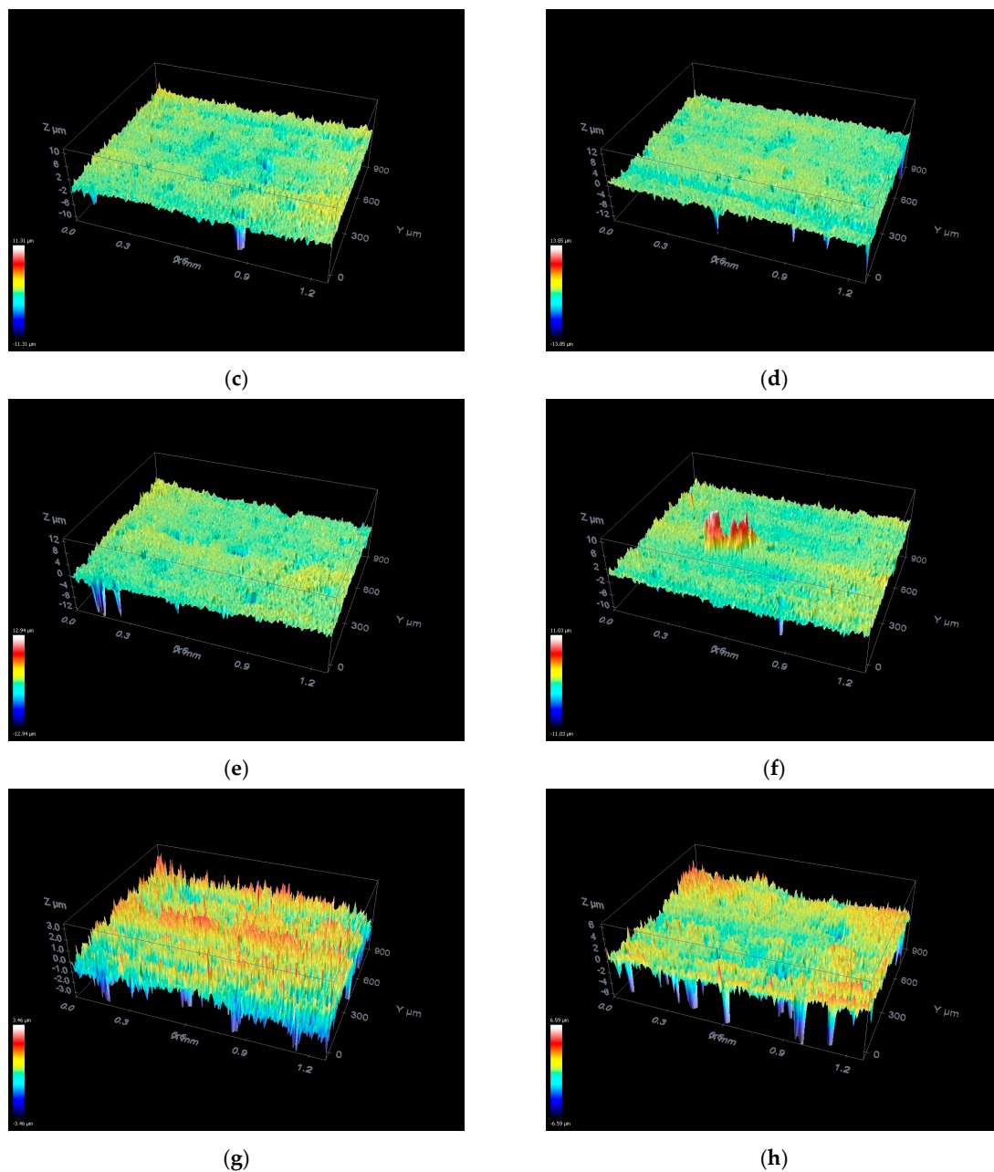
Figure 3. Confocal microscopy: (a) Without cutting; (b) 25 \mu\text{m} ; (c) 35 \mu\text{m} ; (d) 50 \mu\text{m} ; (e) 105 \mu\text{m} ; (f) 150 \mu\text{m} ; (g) 210 \mu\text{m} ; and (h) 350 \mu\text{m} .
