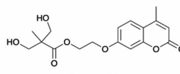
Coumarin diol
