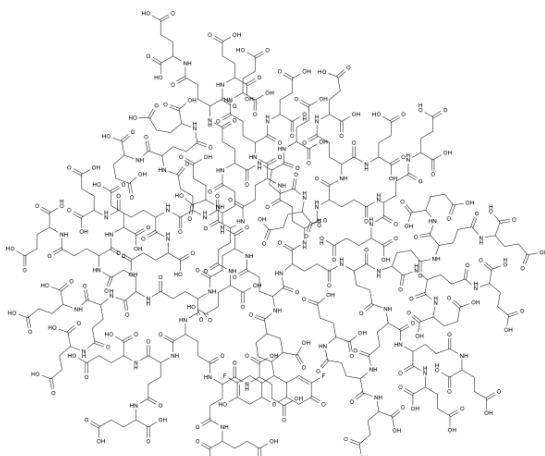
NBD-PG-LYS-G4
