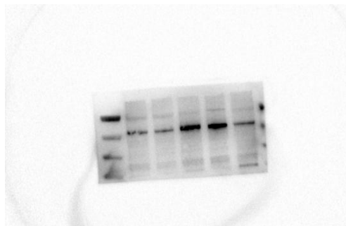
WTAP
