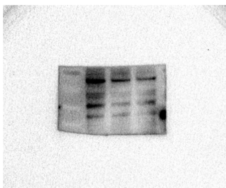
siMETTL3-BMI1
