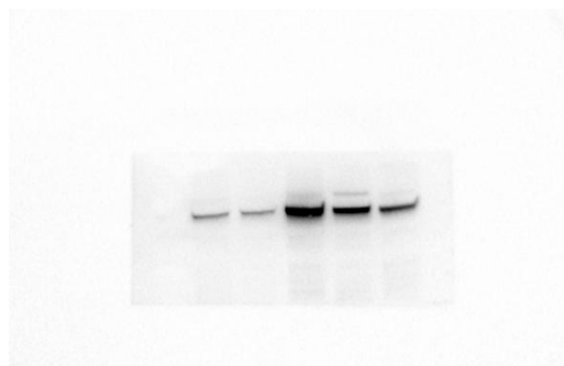
FTO
