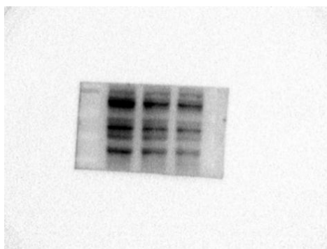
siMETTL3-OCT4
