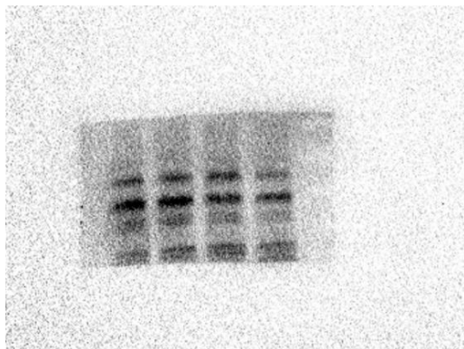
siSALL4-BMI1
