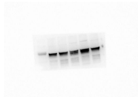
ALKBH5
