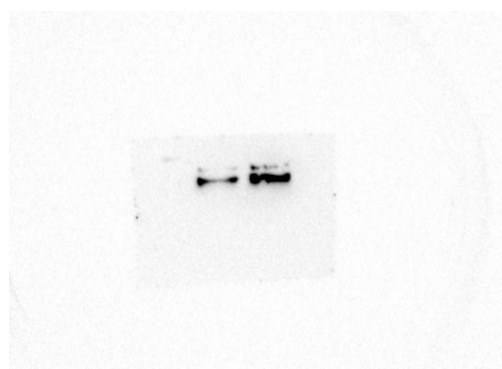
OE-SALL4-BMI1
