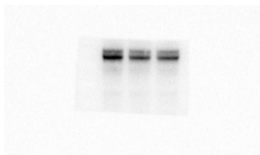
siMETTL3-c-MYC
