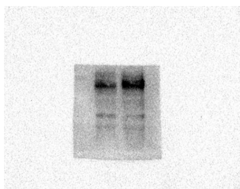
OE-METTL3-Nanog
