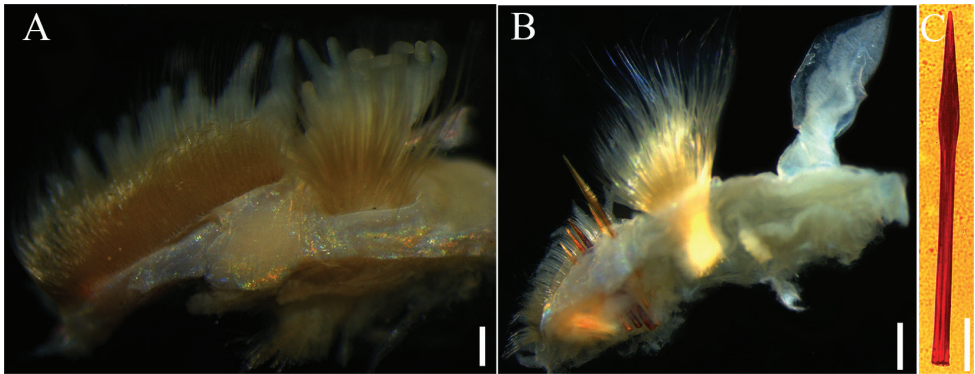
Figure 6. Phylo fimbriata (Moore, 1903) A anterior thoracic chaetiger, anterior view B posterior thoracic chaetiger, anterior view C modified spines. Scale bars: 0.5 mm ( B, C ); 0.2 mm ( A ).
