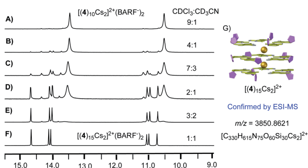
Fig. 6 ^1\text{H} NMR spectra of \text{CD}_3\text{CN} titration experiments using [(4)_{10}\text{Cs}_2]^{2+}(\text{BARF}^-)_2 (A) \text{CDCl}_3 : \text{CD}_3\text{CN} = 9 : 1 ; (B) \text{CDCl}_3 : \text{CD}_3\text{CN} = 4 : 1 ; (C) \text{CDCl}_3 : \text{CD}_3\text{CN} = 7 : 3 ; (D) \text{CDCl}_3 : \text{CD}_3\text{CN} = 2 : 1 ; (E) \text{CDCl}_3 : \text{CD}_3\text{CN} = 3 : 2 ; (F) \text{CDCl}_3 : \text{CD}_3\text{CN} = 1 : 1 ; (G) model of \text{isoG}_{15} formed.
