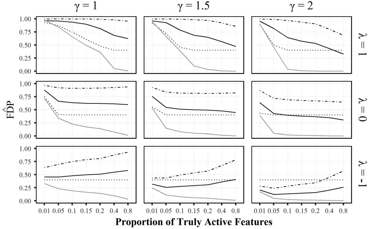
--- FDP Bound — mFDP ..... FDP fbH -.- True FDP
