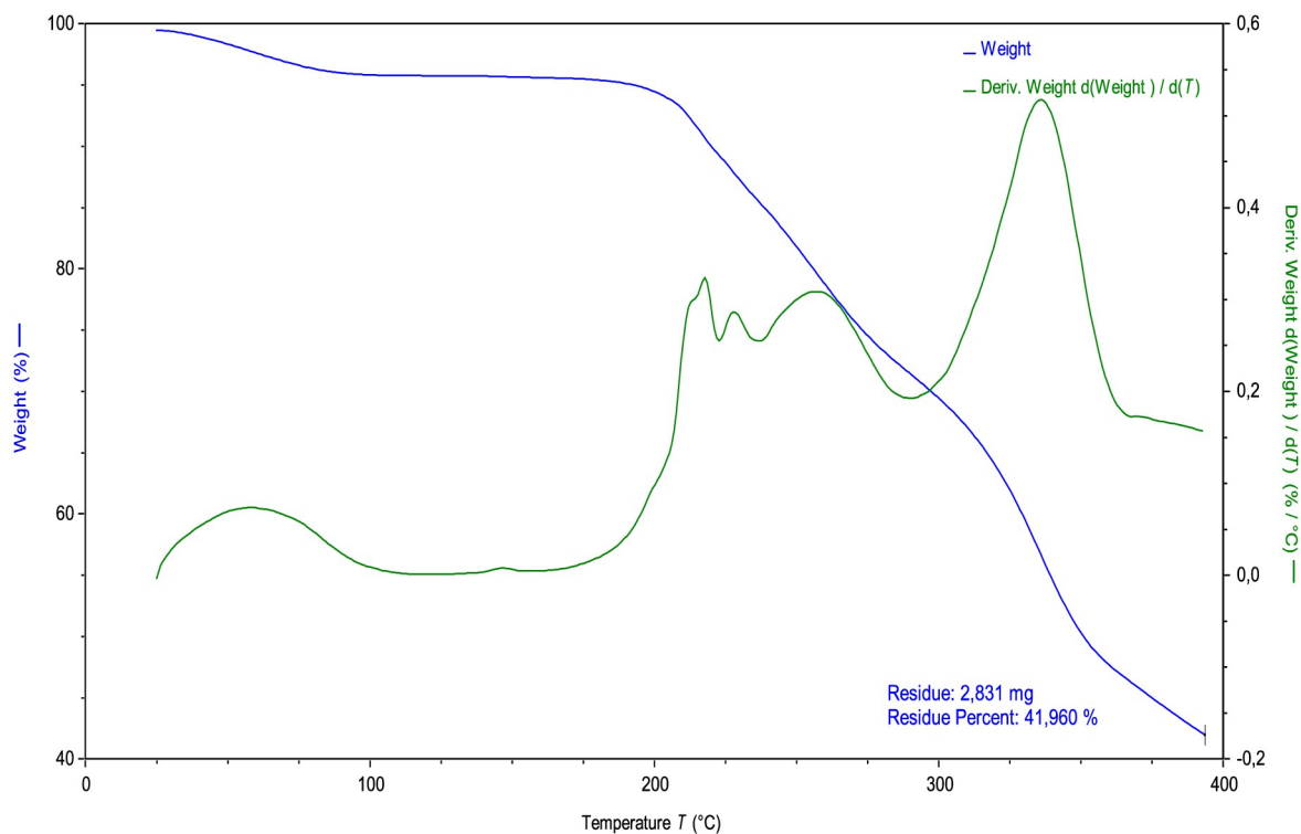
Fig 7. TGA rosuvastatin calcium.
