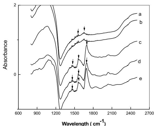
Figure 5 FTIR spectra of \text{Fe}_3\text{O}_4@Au (a), \text{Fe}_3\text{O}_4 -LAA (b) huPrPrec (c), \text{Fe}_3\text{O}_4@Au -huPrPrec (d) \text{Fe}_3\text{O}_4 -LAA-huPrPrec (e).
