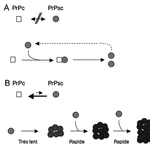
Fig. 1 – Modèles de la conversion de la PrP c en PrP sc [61,62]. A. Modèle de polymérisation assistée par une amorce. B. Modèle de nucléation-polymérisation.
