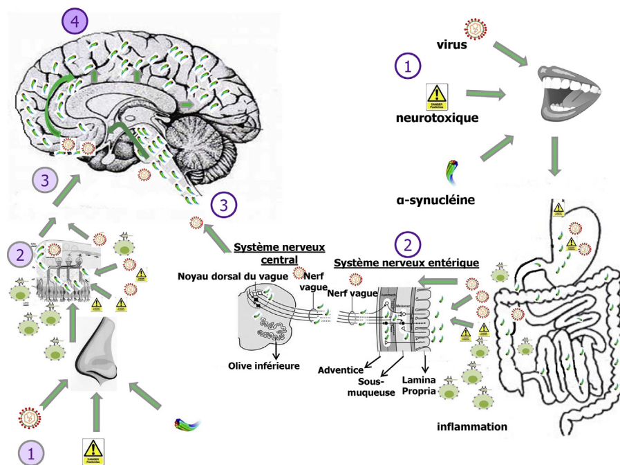
Fig. 3 – Représentation schématique des possibles facteurs responsables de l'agrégation et de la propagation de l' \alpha -synucléine selon un mécanisme prion-like. 1 – Entrée d'un facteur exogène (virus, neurotoxique, agrégats d' \alpha -synucléine) par voie orale ou nasale, éventuellement favorisée par un phénomène inflammatoire. 2 – Dissémination des agrégats d' \alpha -synucléine ingérés, inhalés ou formés, in situ, sous l'influence du virus ou du neurotoxique à partir du système nerveux périphérique. L'hypothèse alternative serait la propagation directe d'un virus dont la réplique périphérique ou centrale entraînerait l'agrégation de l' \alpha -synucléine le long de son trajet. 3 – Accumulation de l' \alpha -synucléine dans le tronc cérébral (voie digestive) ou dans le lobe temporal (voie olfactive). 4 – Propagation des agrégats d' \alpha -synucléine à l'ensemble du cortex.
