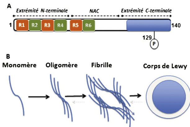
Fig. 2 – A. Structure primaire de l' \alpha -synucléine humaine. L' \alpha -synucléine humaine est une petite protéine de 140 acides aminés divisée d'un point de vue fonctionnel en 3 domaines. La partie amino-terminale (résidus 1 à 60) contient 6 domaines de répétition imparfaite (R1 à R6) contenant des résidus lysine, impliqués dans la liaison aux lipides et aux membranes cellulaires. Le domaine central (résidus 61 à 95) joue un rôle essentiel dans les capacités d'agrégation de la protéine alors que l'extrémité carboxy-terminale (résidus 96–140) serait responsable de l'activité et contient le principal sites de phosphorylation sur le résidu sérine 129. B. Agrégation de l' \alpha -synucléine. Des études in vitro ont montré que l' \alpha -synucléine est en équilibre dynamique. La forme monomérique a une capacité naturelle à s'agréger en structures amyloïdes grâce à son domaine central selon la progression suivante : dimères, oligomères, protofibrilles et fibrilles puis enfin corps de Lewy.
