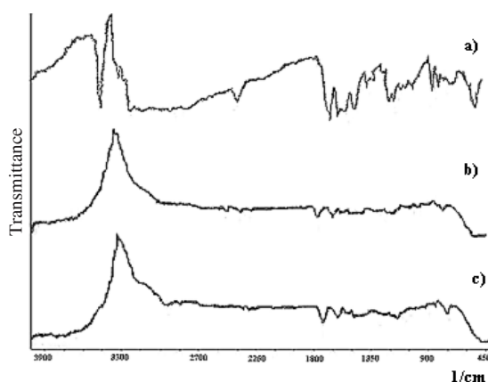
Figure 1. FT-IR spectra: a) LMG, b) LMG+E-RSPO c) LMG+E-RLPO
