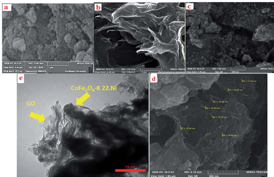
Fig. 8 SEM images of \text{CoFe}_2\text{O}_4 (a), GO (b), \text{CoFe}_2\text{O}_4@\text{GO} (c), \text{CoFe}_2\text{O}_4@\text{GO}-\text{K} 22 \cdot \text{Ni} (d) and TEM image of \text{CoFe}_2\text{O}_4@\text{GO}-\text{K} 22 \cdot \text{Ni} (e).
