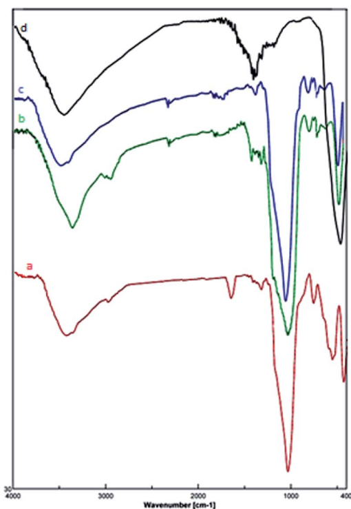
Fig. 2 FT-IR spectra of (a) \text{Fe}_3\text{O}_4@SiO_2@(CH_2)_3OCO_2Na , (b) \text{Fe}_3\text{O}_4@SiO_2(CH_2)_3Cl , (c) \text{Fe}_3\text{O}_4@SiO_2 , and (d) \text{Fe}_3\text{O}_4 MNPs.
