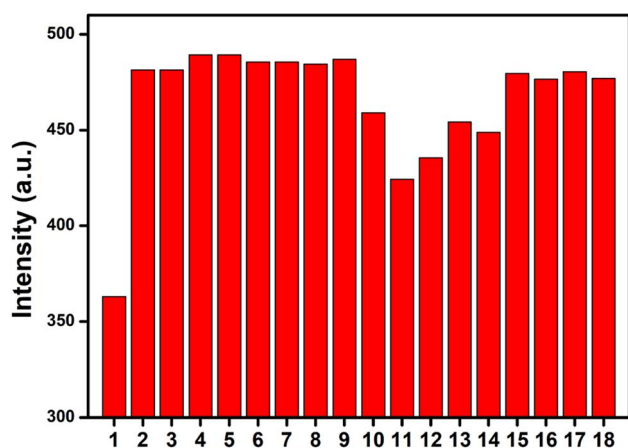
Fig. 6 Anti-interference experiment of CIT-Z for detecting \text{CN}^- (1) blank; (2) \text{CN}^- ; (3) \text{Na}^+ ; (4) \text{K}^+ ; (5) \text{SO}_4^{2-} ; (6) \text{CH}_3\text{COO}^- ; (7) \text{Zn}^{2+} ; (8) \text{HPO}_4^{2-} ; (9) \text{HCO}_3^- ; (10) \text{H}_2\text{PO}_4^{2-} ; (11) \text{CO}_3^{2-} ; (12) \text{Cl}^- ; (13) \text{Fe}^{3+} ; (14) \text{Fe}^{2+} ; (15) \text{Co}^{2+} ; (16) \text{Hg}^{2+} ; (17) \text{Ni}^+ ; (18) \text{Mg}^{2+} ).
