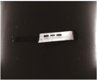
NAT10
