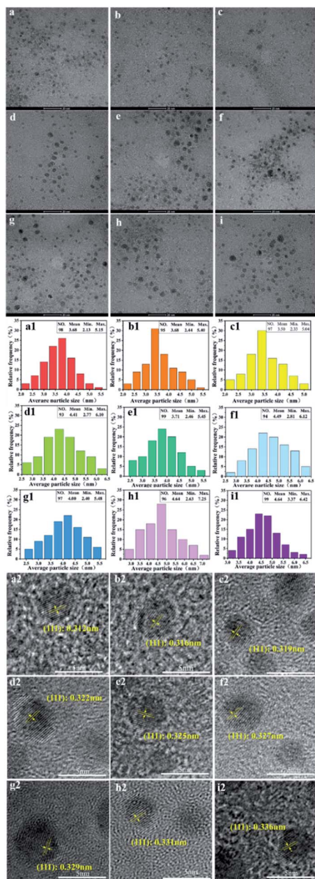
Fig. 3 TEM, HRTEM and size distribution of the SRB-derived ternary Zn_xCd_{1-x}S alloyed QDs at different molar ratios of Cd/Zn. TEM of Cd/Zn = 0 : 1 (a), 1 : 50 (b), 1 : 40 (c), 1 : 30 (d), 1 : 20 (e), 1 : 15 (f), 1 : 9 (g), 1 : 5 (h), 1 : 0 (i); the particle size distribution of Cd/Zn = 0 : 1 (a1), 1 : 50 (b1), 1 : 40 (c1), 1 : 30 (d1), 1 : 20 (e1), 1 : 15 (f1), 1 : 9 (g1), 1 : 5 (h1), 1 : 0 (i1); HRTEM images of Cd/Zn = 0 : 1 (a2), 1 : 50 (b2), 1 : 40 (c2), 1 : 30 (d2), 1 : 20 (e2), 1 : 15 (f2), 1 : 9 (g2), 1 : 5 (h2), 1 : 0 (i2).
