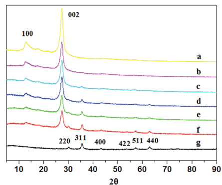
Fig. 2 XRD patterns of (a) pure g\text{-C}_3\text{N}_4 , (b) \text{FeOCN-2} , (c) \text{FeOCN-4} , (d) \text{FeOCN-6} , (e) \text{FeOCN-8} , (f) \text{FeOCN-10} , (g) pure \text{Fe}_3\text{O}_4 .
