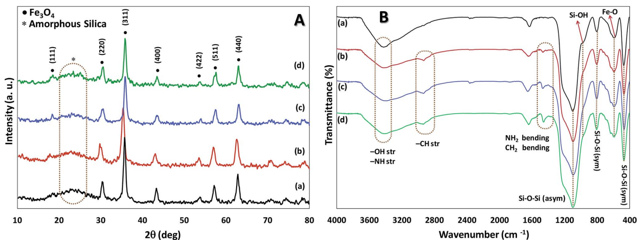
Fig. 1 (A) The XRD pattern, (B) the FTIR spectra of \text{Fe}_3\text{O}_4@SiO_2 (a), \text{Fe}_3\text{O}_4@SiO_2\text{-APTES} (b), \text{Fe}_3\text{O}_4@SiO_2\text{-APTES-H}_2\text{L}^{\text{GDC}} (c) and \text{Fe}_3\text{O}_4@SiO_2\text{-APTES-MnL}^{\text{GDC}} (d).
