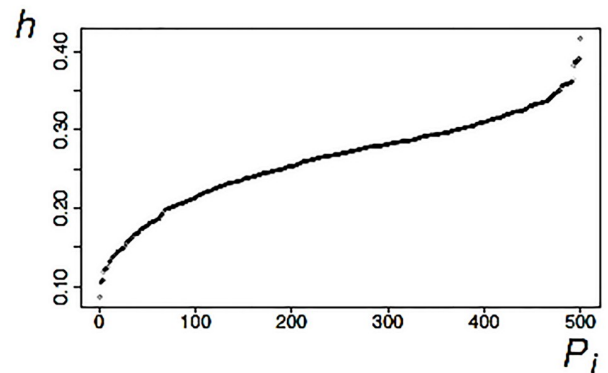
(d) Ranked h distribution versus P_i^{\text{in}} for \mathcal{G}_2^1 .
