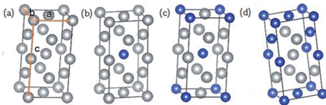
Fig. 1 Crystal structures of (a) Ag, (b) Cu 0.125 Ag 0.875 , (c) Cu 0.25 Ag 0.75 , (d) Cu 0.5 Ag 0.5 .
