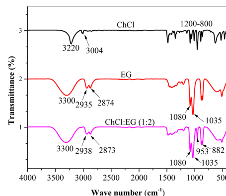
Fig. 1 ChCl : EG (1 : 2) DES confirmation via FT-IR spectra.
