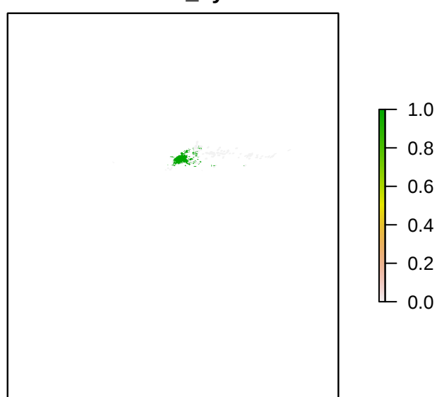
S2Colias_hyale
