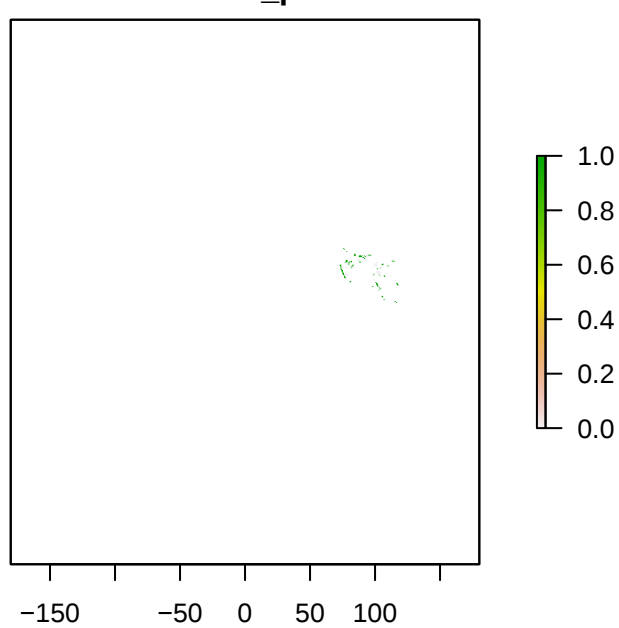
S4Moduza_procris
