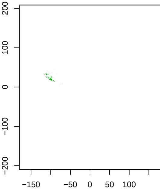
S3Eurema_mexicana
