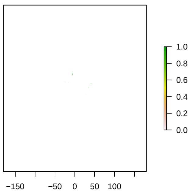
S4Borbo_borbonica
