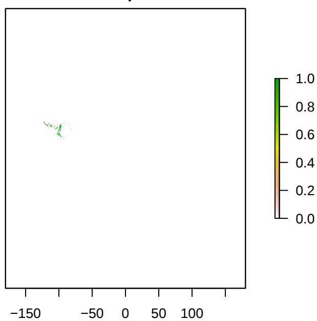
S4Pontia_protodice
