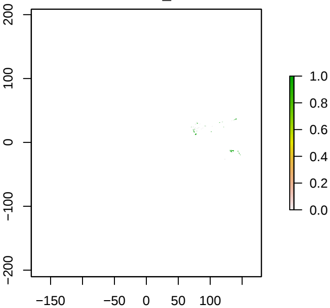
S3Eurema_laeta
