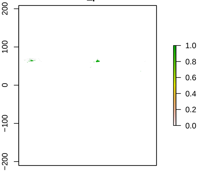
S1Colias_palaeno
