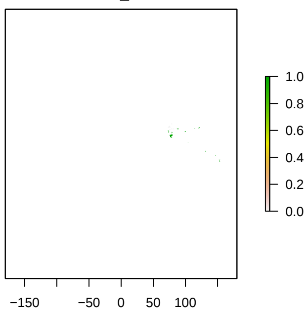
S4Hasora_chromus
