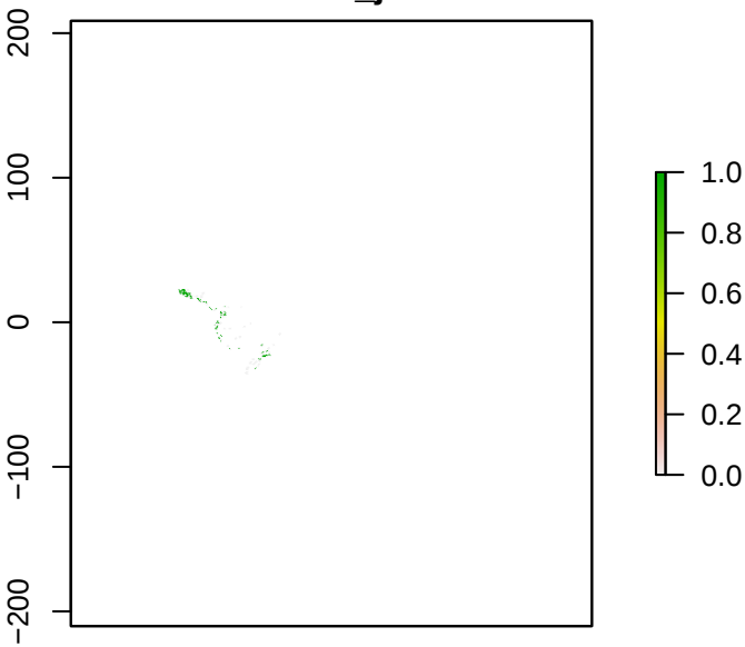
S1Dione_juno
