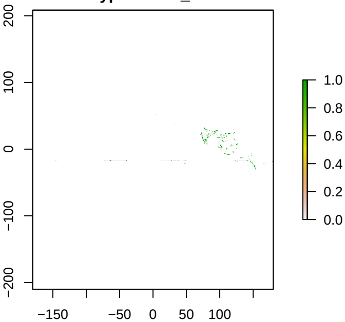
S3Hypolimnas_bolina
