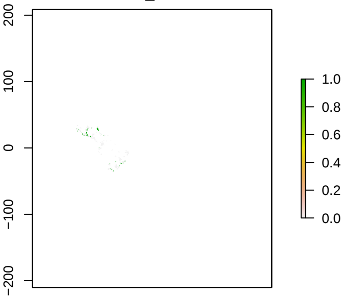
S1Ascia_monuste
