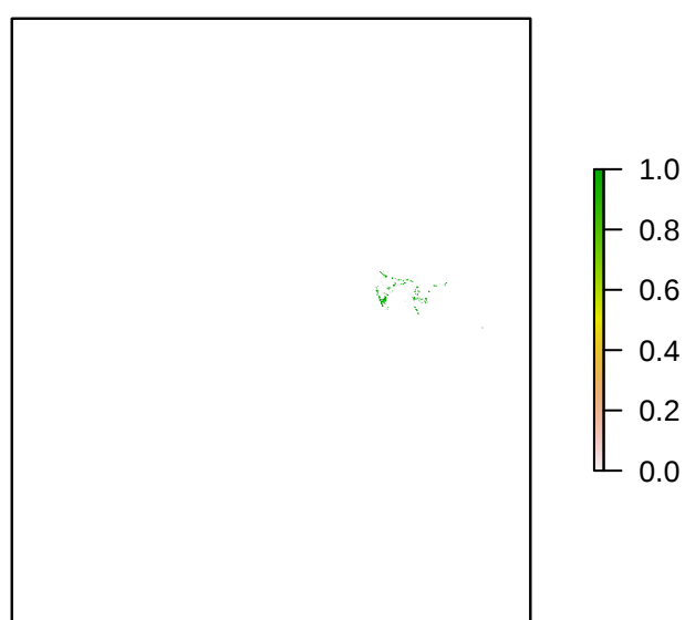
S2Junonia_lemonias
