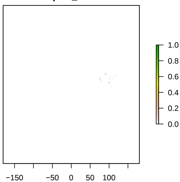
S4Papilio_helenus
