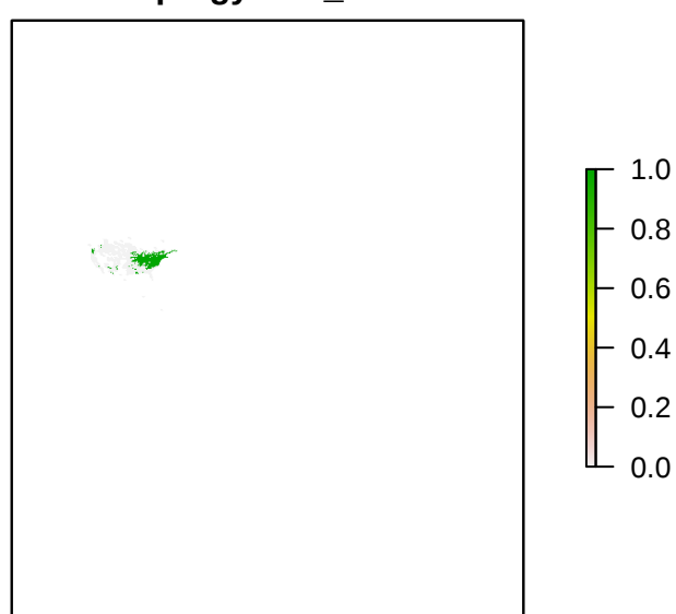
S2Epargyreus_clarus
