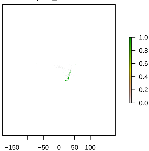
S4Papilio_demodocus
