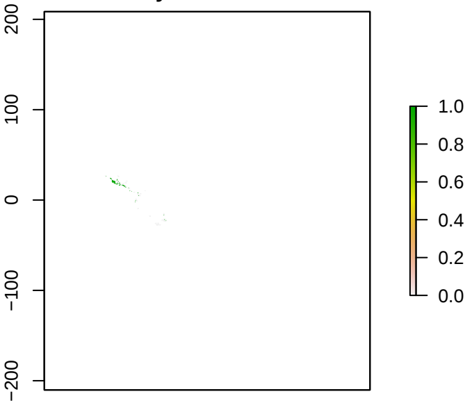
S1Smrna_blomfildia
