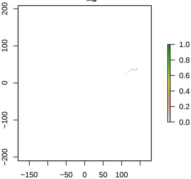
S3Parnara_guttatus
