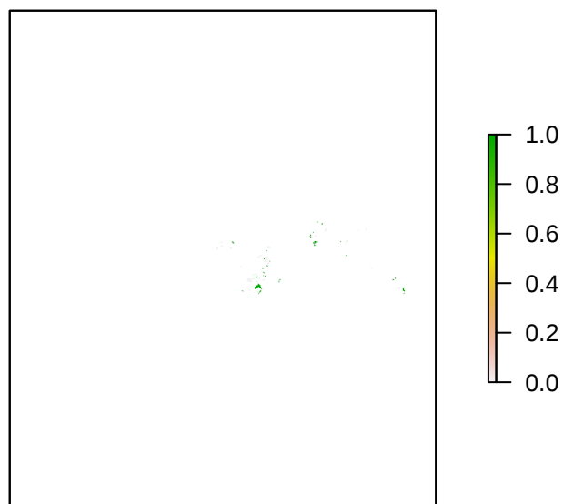
S2Eurema_brigitta
