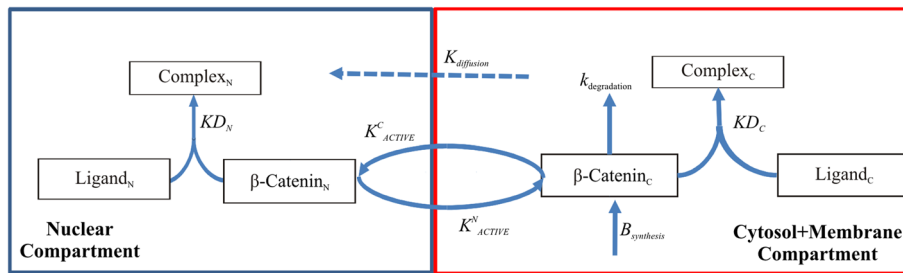
(b) Tan
