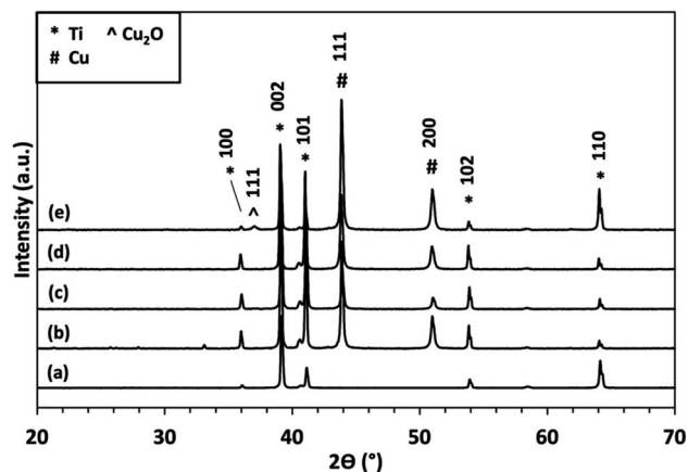
Fig. 3 XRD patterns of (a) NT-Control, (b) Ti/Cu 60, (c) NT/Cu 30, (d) NT/Cu 60, and (e) NT/Cu 90.
