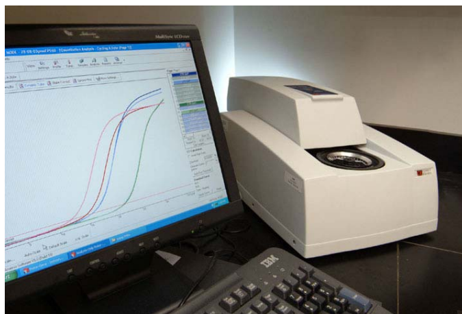
Fig. 1: The Rotor-Gene 3000 apparatus.
