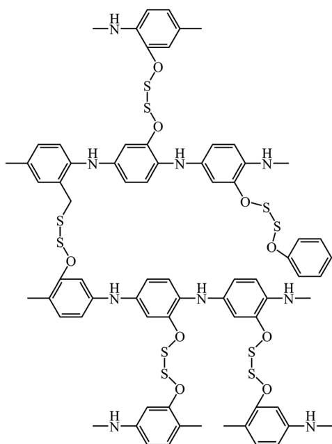
Fig. 2 Poly[bis(2-aminophenoxy)disulfide].
