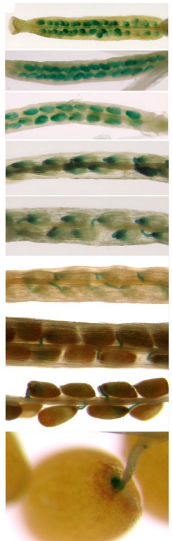
AtbZIP2
