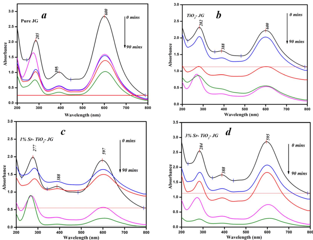
Fig. 9 Absorption spectra of (a) JG (b) \text{TiO}_2 -JG (c) 1% \text{Sr-TiO}_2 -JG (d) 3% \text{Sr-TiO}_2 -JG.
