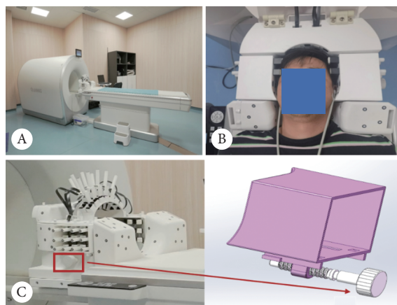
图1 OPM-MEG设备
