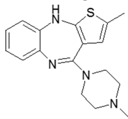
Olanzapine
