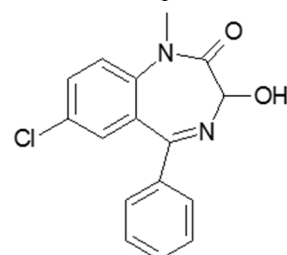
Temazepam
