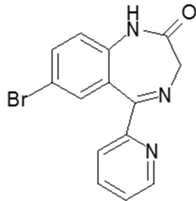
Bromazepam
