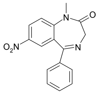
Nimetazepam
