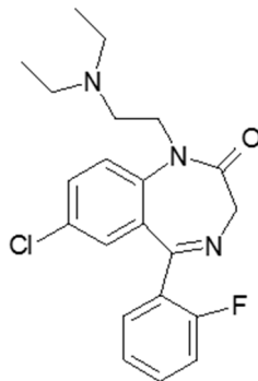
Flurazepam
