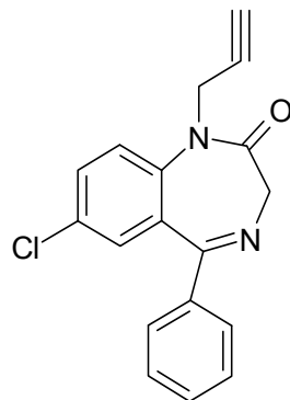
Pinazepam
