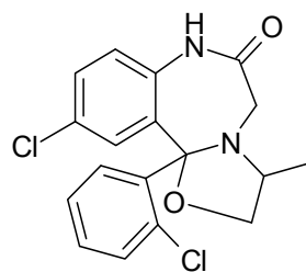
Mexazolam
