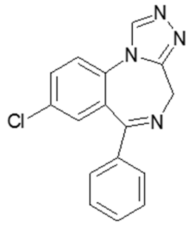
Estazolam
