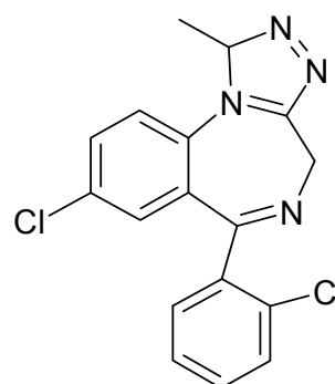
Triazolam
