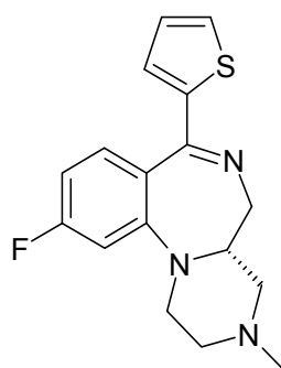
Timelotem
