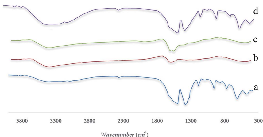
Fig. 3 FTIR spectra for synthesized samples (a) UIO-66, (b) \text{MnFe}_2\text{O}_4 , (c) \text{MnFe}_2\text{O}_4\text{-TiO}_2 , (d) \text{UIO-66-MnFe}_2\text{O}_4\text{-TiO}_2 .
