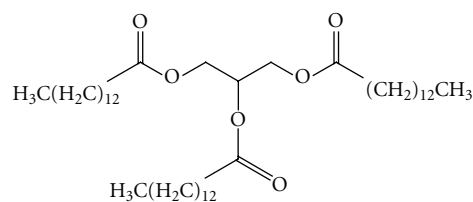
Trimyristin
