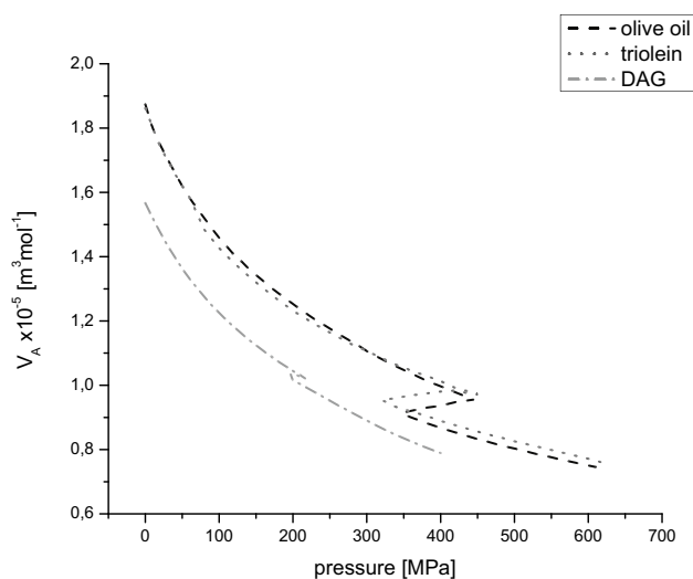
Fig. 9 Parameter V_A vs pressure at 20 °C
