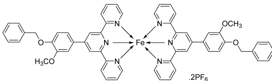
[Fe(4-(Benzyloxy)-3-methoxyphenyl)-2,2':6',2''-terpyridine) 2 ] (PF 6 ) 2
