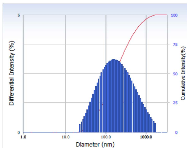
Fig. 4 PSA of La 2 O 3 .
