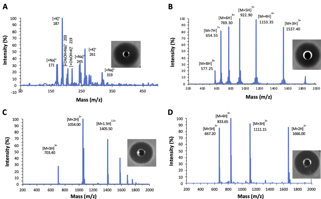
FIG 1 LC/MS and agar well diffusion assay of (A) reuterin, (B) pediocin PA-1, (C) MccJ25, (D) nisin Z.
