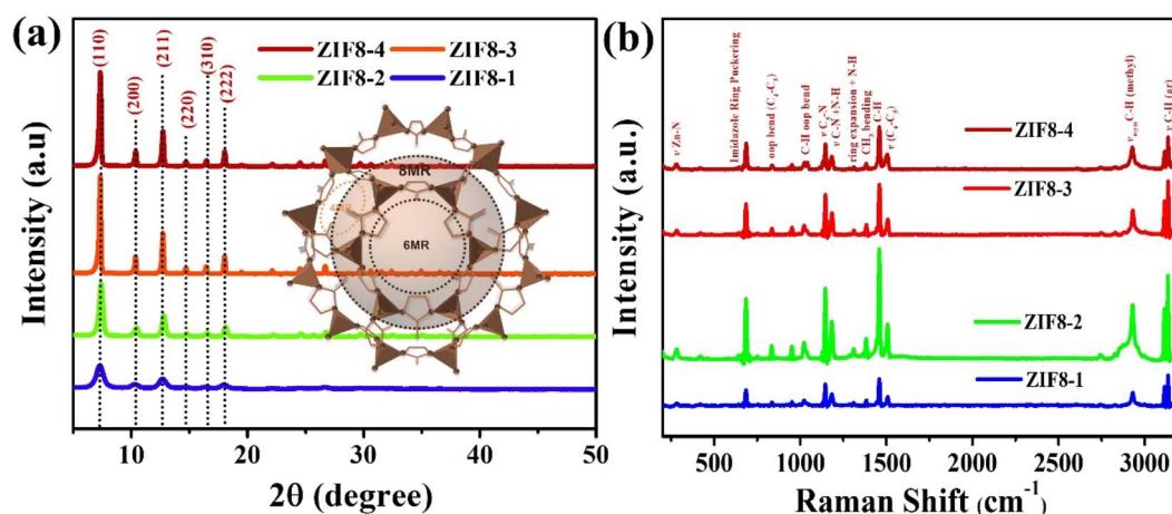
Fig. 3 (a) XRD patterns of the ZIF8-1, ZIF8-2, ZIF8-3 and ZIF8-4 nanocrystals and (b) Raman analysis for the ZIF8-1, ZIF8-2, ZIF8-3 and ZIF8-4 nanocrystals.
