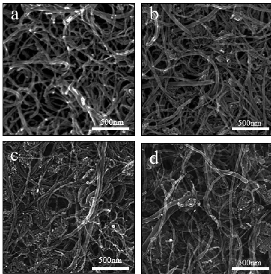
Fig. 6 SEM images of Fe 3 O 4 /MWCNT buckypapers with different m_{\text{Fe}_3\text{O}_4} to m_{\text{MWCNT}} ratios: (a) 0 : 1, (b) 1 : 1, (c) 2 : 1 and (d) 3 : 1.
