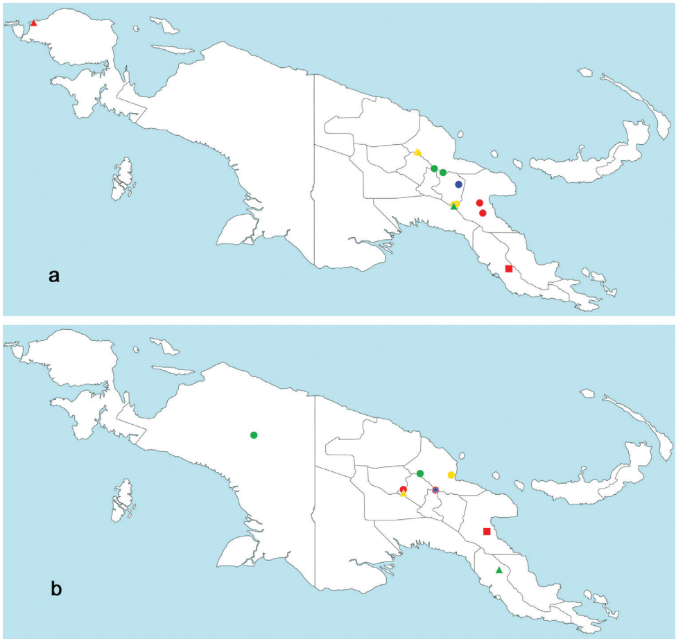
Figure 65. Distribution of Labiobaetis in New Guinea: a red circle, L. tuberculatus ; yellow circle, L. branchiaesetis sp. n.; green circle, L. magnovaldus sp. n.; red triangle, L. planus sp. n.; blue circle, L. podolakae sp. n.; yellow triangle, L. rutschmannae sp. n.; green triangle, L. schwanderae sp. n.; red square, L. centralensis sp. n. b yellow circle, L. paravittilis sp. n.; red circle, L. altus sp. n.; green circle, L. gindroi sp. n.; yellow triangle, L. vitilis ; green triangle, L. pindaundensis sp. n.; red square, L. xeniolus ; blue star, L. wilhelmensis sp. n. / L. dendrisetis sp. n. / L. pindaundensis sp. n.
