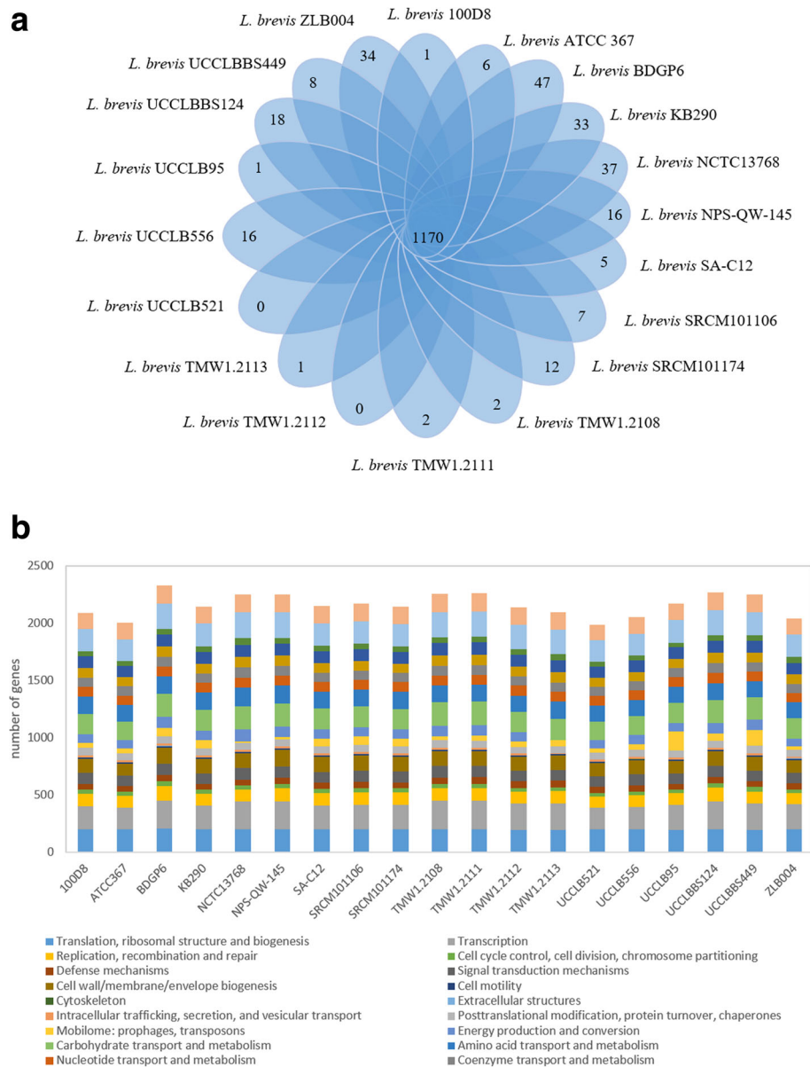
Fig. 4 Comparative genomics of chromosomal orthologous proteins in L. brevis . Panel a: Venn diagram representing the orthologous and unique gene families of 19 L. brevis strains obtained by MCL clustering. Panel b: Cluster of Orthologous Groups (COG) classification of L. brevis . Histograms represent COG predictions for each of the following 16 L. brevis isolates: L. brevis 100D8, L. brevis ATCC 367, L. brevis BDGP6, L. brevis KB290, L. brevis NCTC13768, L. brevis NPS-QW-145, L. brevis SA-C12, L. brevis SRCM101106, L. brevis SRCM101174, L. brevis TMW 1.2108, L. brevis TMW 1.2111, L. brevis TMW 1.2112, L. brevis TMW 1.2113, L. brevis UCCLB521, L. brevis UCCLB556, L. brevis UCCLB95, L. brevis UCCLBBS124, L. brevis UCCLBBS449, L. brevis ZLB004
