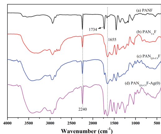
Fig. 1 The FTIR spectra of (a) PANF, (b) PAN TAF , (c) PAN QA-C4 F and (d) PAN QA-C4 F-Ag(0).
